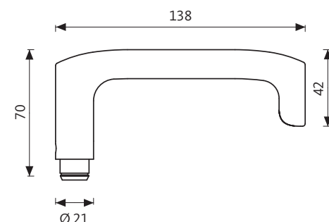
DIRIGENT H7.0
