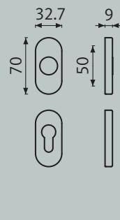
Ovaal rozet
