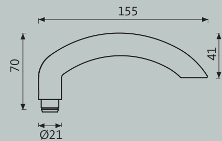
LEGATO H5.0
