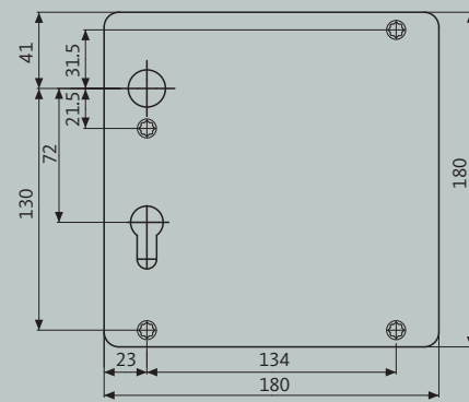
Breedschild
