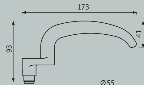
TREMOLO H6.0
