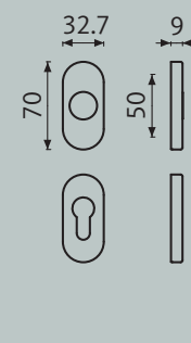
Ovaal rozet
