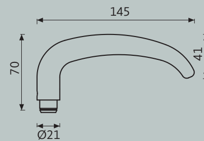
TREMOLO H6.0
