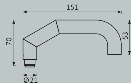
RONDO H1.1
