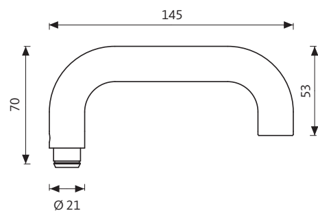
RONDO H1.0
