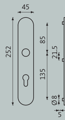
Langschild
