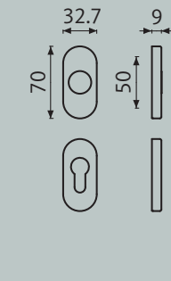
Ovaal rozet
