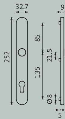
Smalschild
