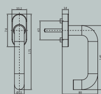
Raamkruk
