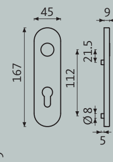
Kortschild
