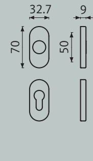
Ovaal rozet
