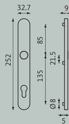
Smalschild
