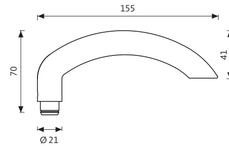
LEGATO H5.0
