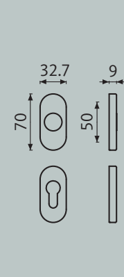
Ovaal rozet
