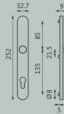
Smalschild
