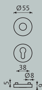
Rozet
