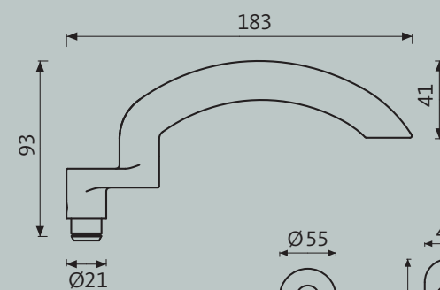
LEGATO H5.2
