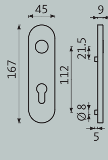
Kortschild
