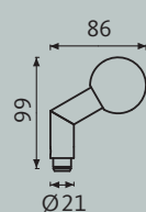
Bolknop K2.1
