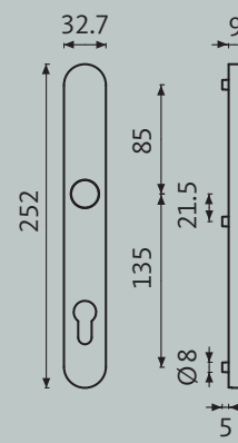
Smalschild
