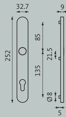
Smalschild
