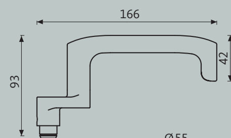
DIRIGENT H7.0
