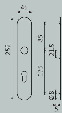
Langschild
