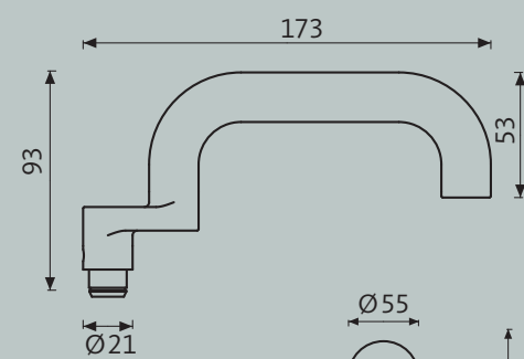
RONDO H1.2
